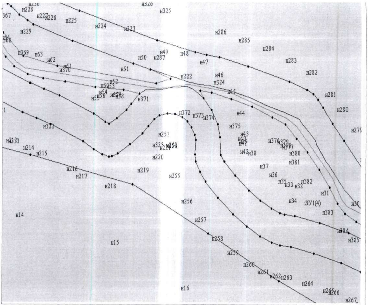
Масштаб 1:500
